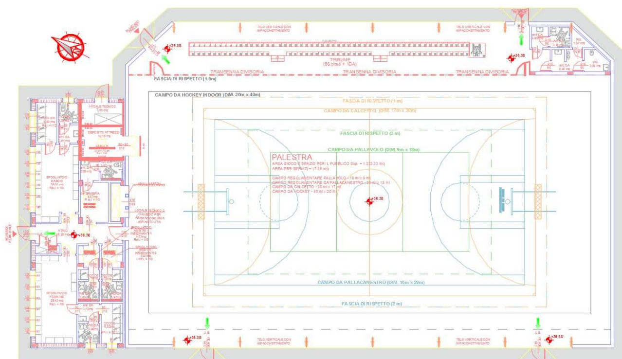
Estratto della tav. A4 – Pianta della palestra e degli spogliatoi
