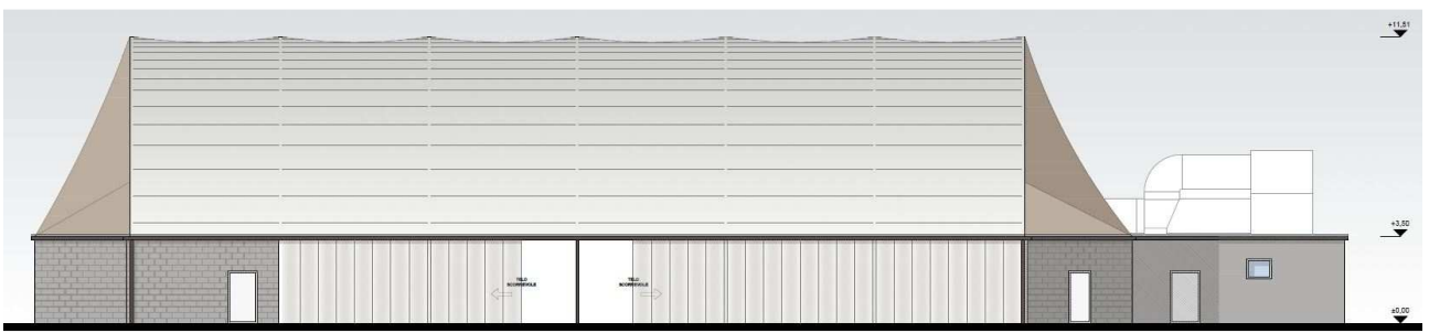
Estratto della tav. A6 – Prospetto nord – est
