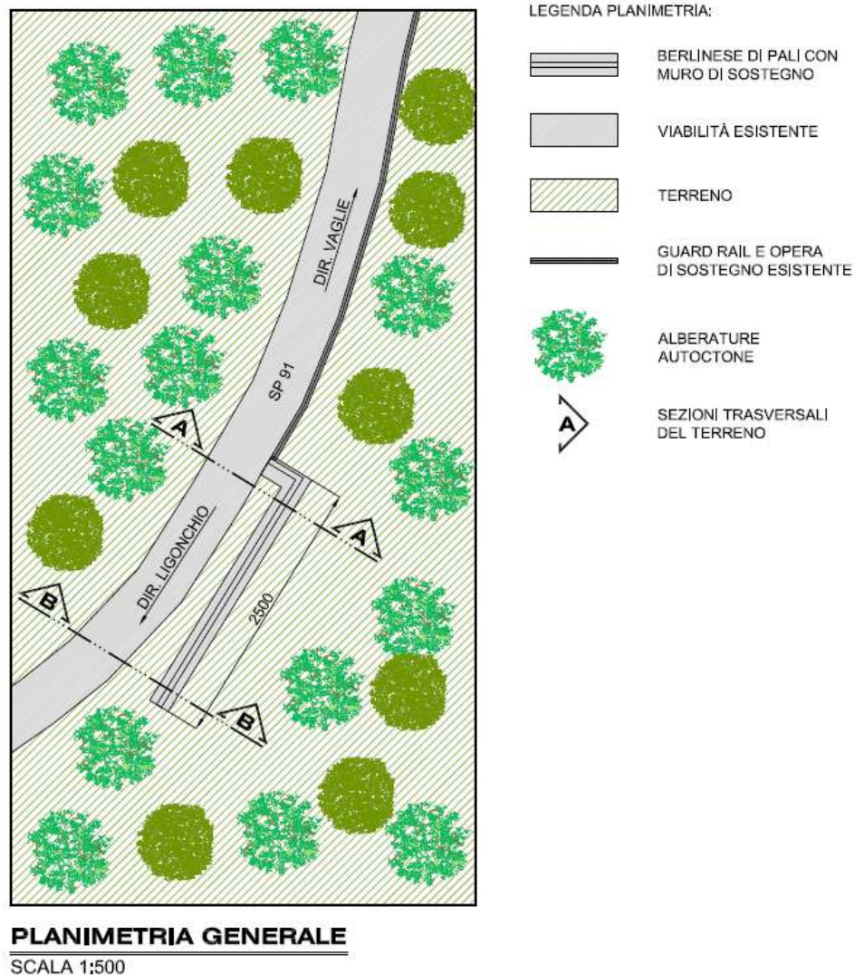
Figura 5 – Estratto della planimetria d'intervento, dove è indicata la posizione dell'opera di consolidamento/sostegno.
