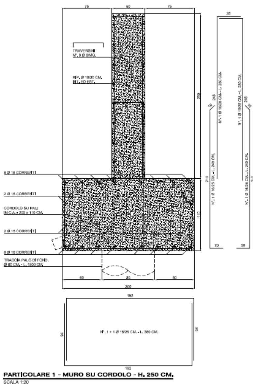
Figura 7 – Sezione tipo del cordolo di collegamento dei pali con la parete del muro di sostegno
