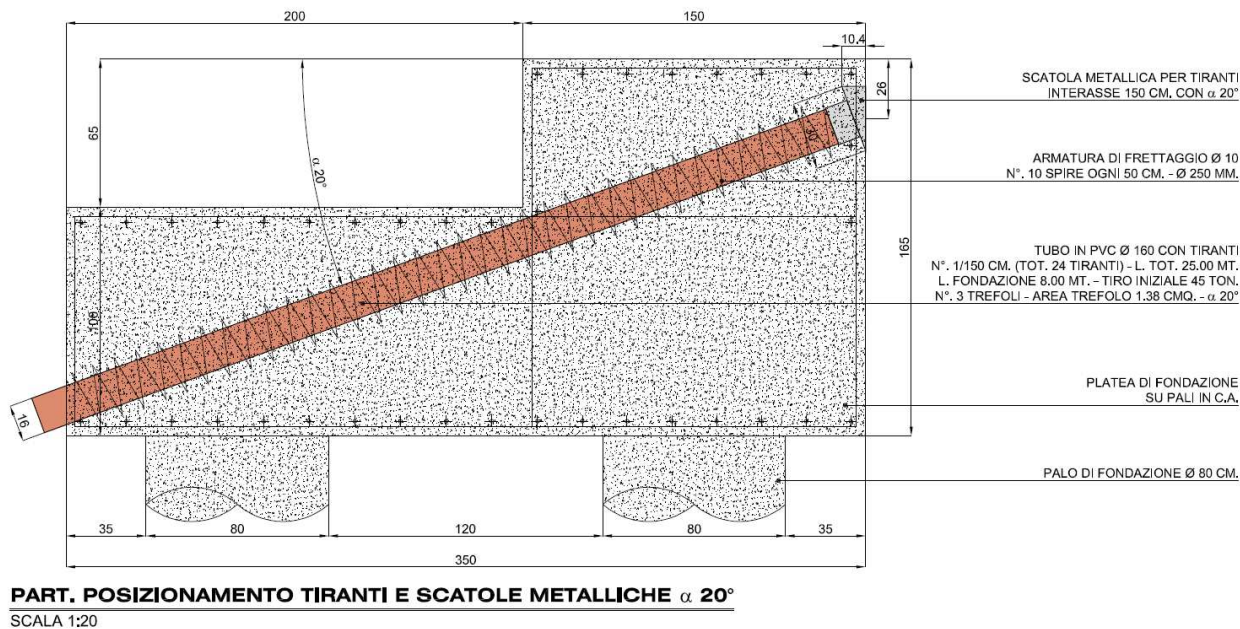
Figura 6 – Particolare della posizione di tiranti in corrispondenza della platea di collegamento dei pali
