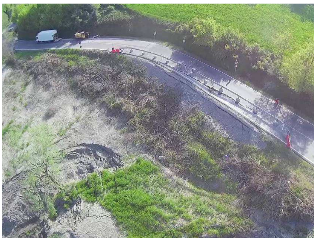
Foto 2 – Particolare del coronamento della frana che interessa la SP 9 al km 10+000.
