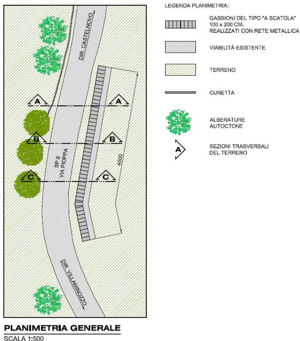
Figura 4 – Estratto della planimetria d'intervento, dove è indicata la posizione dell'opera di consolidamento/sostegno.
