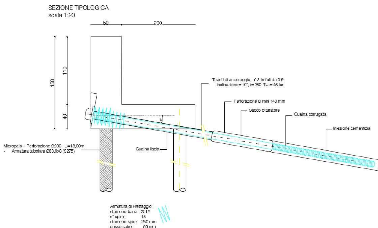
Figura 4 – Sezione tipo dei pali e della trave dell'opera di consolidamento.
