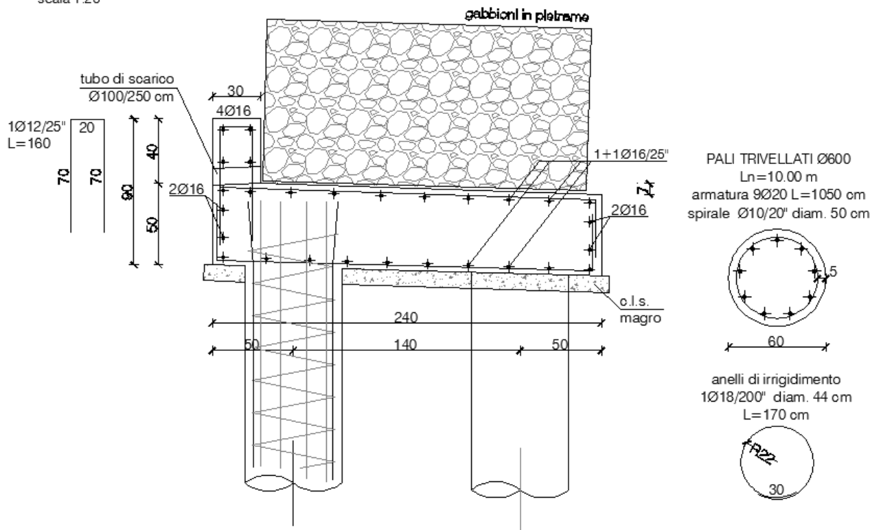
Figura 3 – Sezione tipo dell'opera di consolidamento
