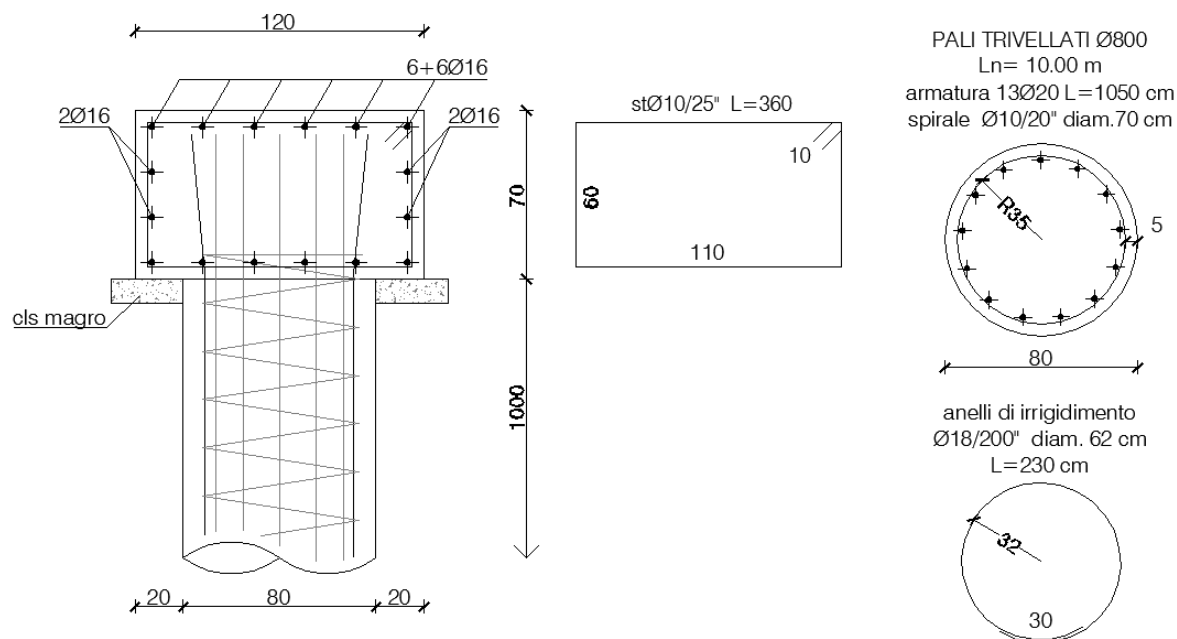
Figura 3 – Sezione tipo dell'opera di consolidamento
