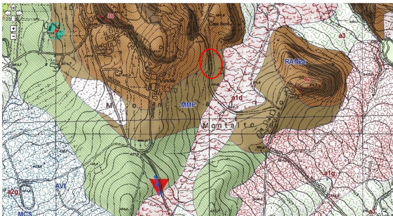
Figura 3- Estratto della Cartografia Geologica della Regione Emilia-Romagna, per l'area interessata dal dissesto sulla SP 74 al km 3+000.
