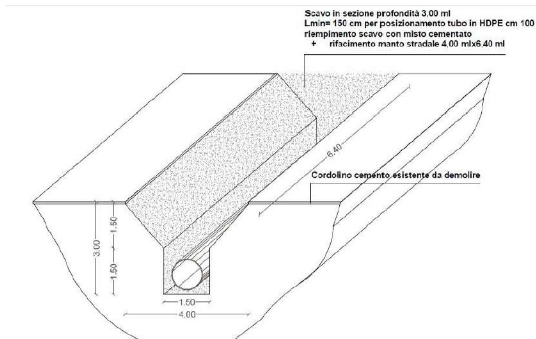
Figura 5 – Esploso assonometrico dello scavo di sbancamento per il posizionamento del nuovo attraversamento idraulico
