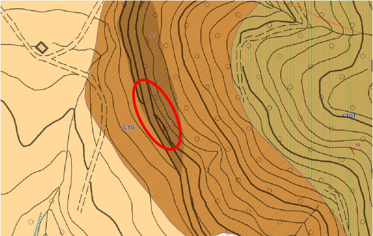
Figura 3 - Estratto della Cartografia Geologica della Regione Emilia-Romagna, per l'area interessata dall'intervento.
