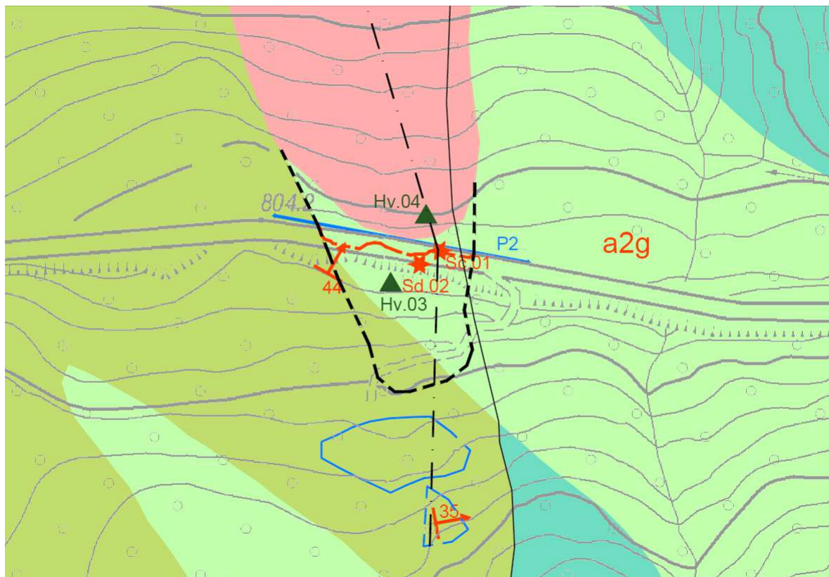
Figura 2 – Ubicazione indagini geognostiche
