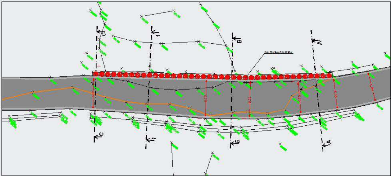
Figura 3 – Estratto della planimetria di intervento di Tav. 11.
