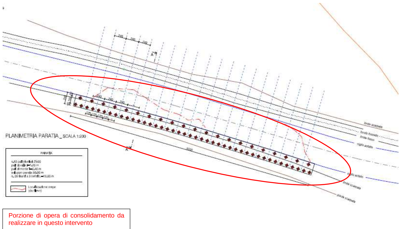
Figura 3 – Estratto della planimetria di intervento.
