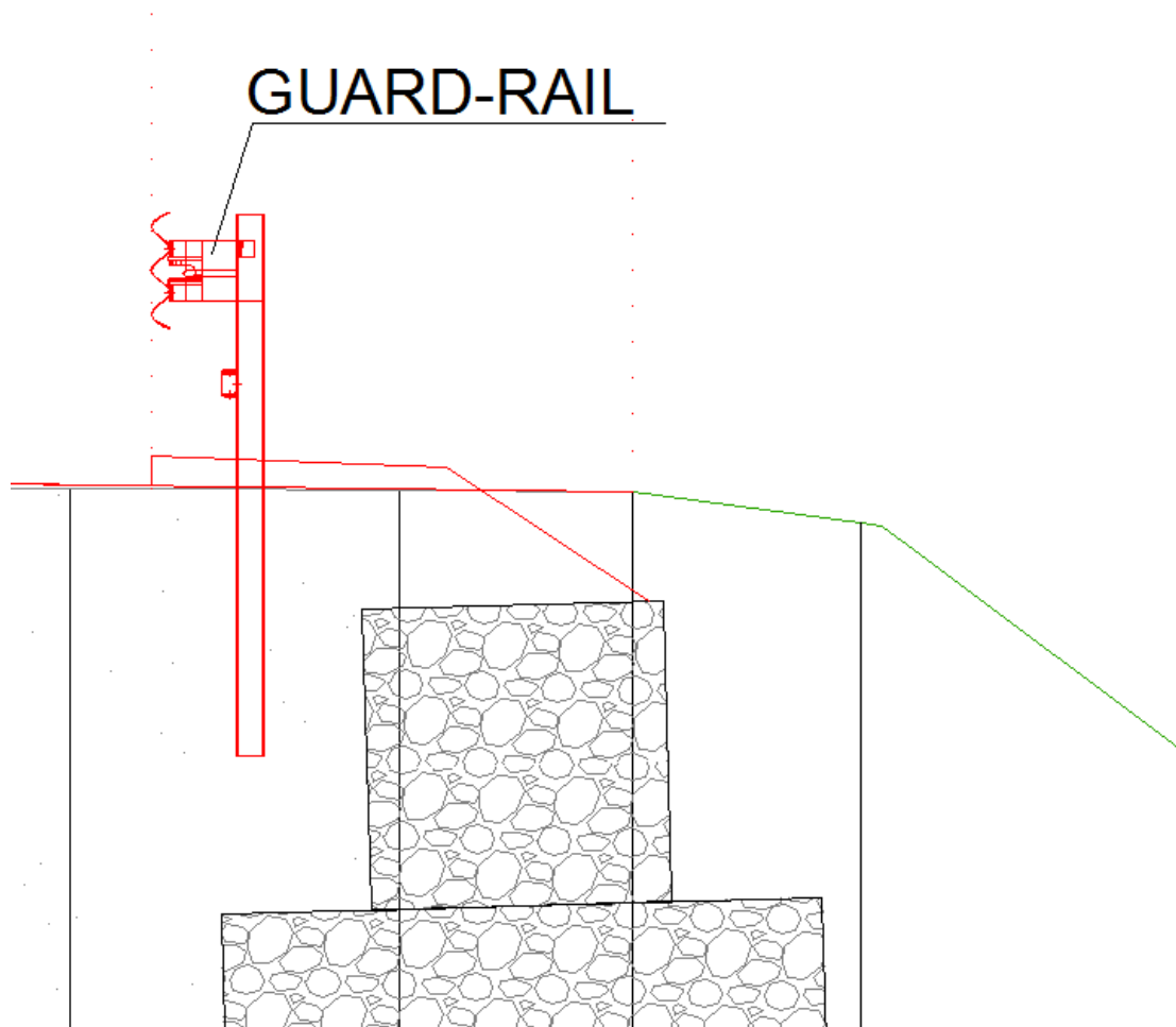
Figura 5 – Sezione tipo della Barriera Bordo laterale sull'arginello
