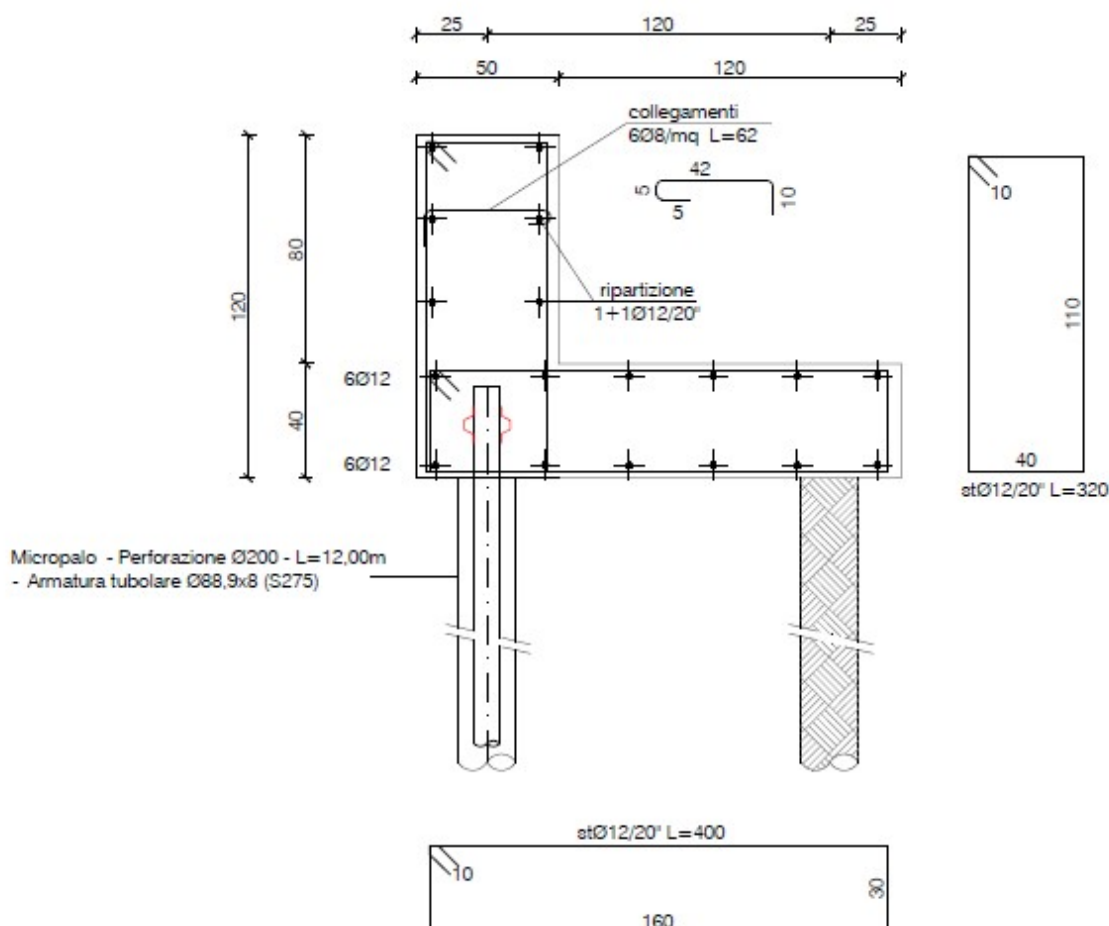
Figura 3 – Sezione tipo dell'opera di consolidamento di valle.
