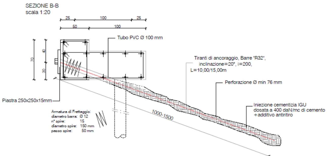
Figura 4 – Sezione tipo dell'opera di consolidamento di monte.
