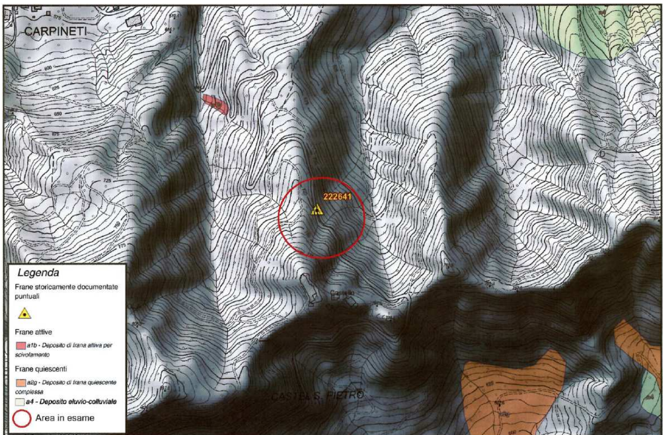
Figura 1 – Estratto di C.T.R. dell'area oggetto di intervento lungo la S.P.76 al km. 1+600.
