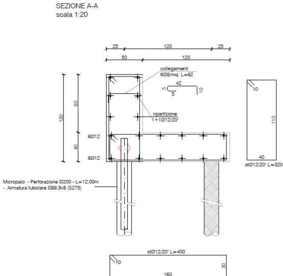
Figura 5 – Sezione tipo dell'opera di consolidamento di valle.
