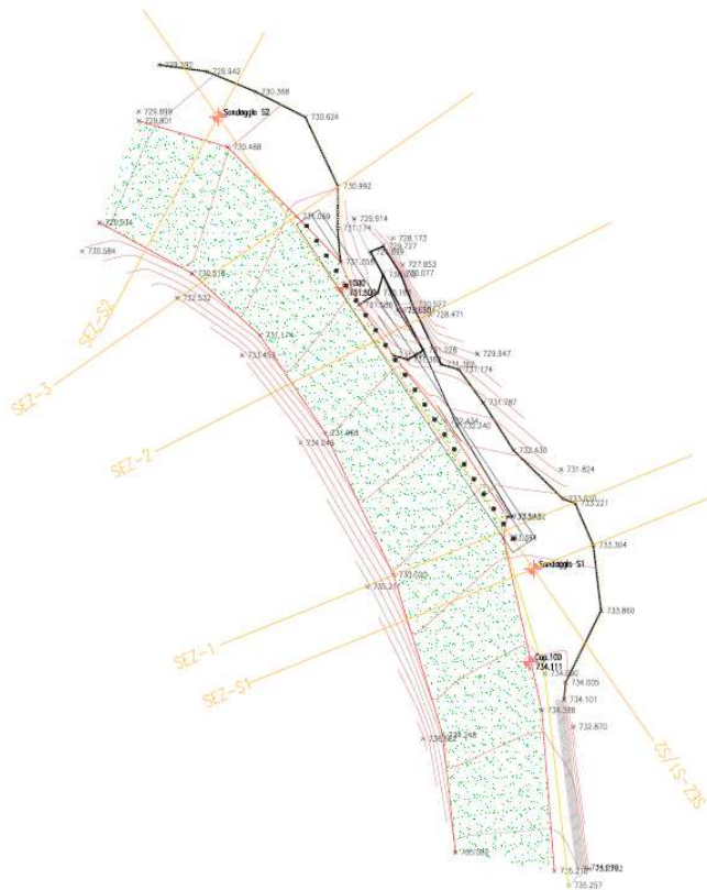
Figura 3 - Estratto della planimetria di intervento.
