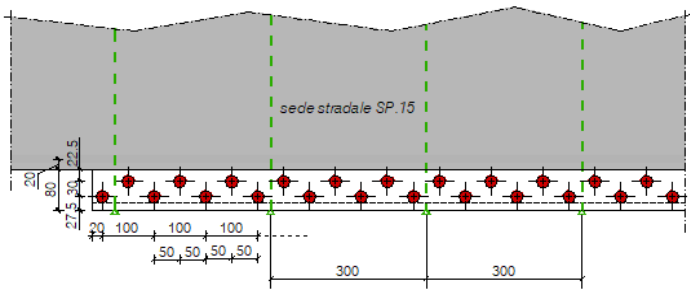
PIANTA BERLINESE (quota sede stradale) scala 1:100
