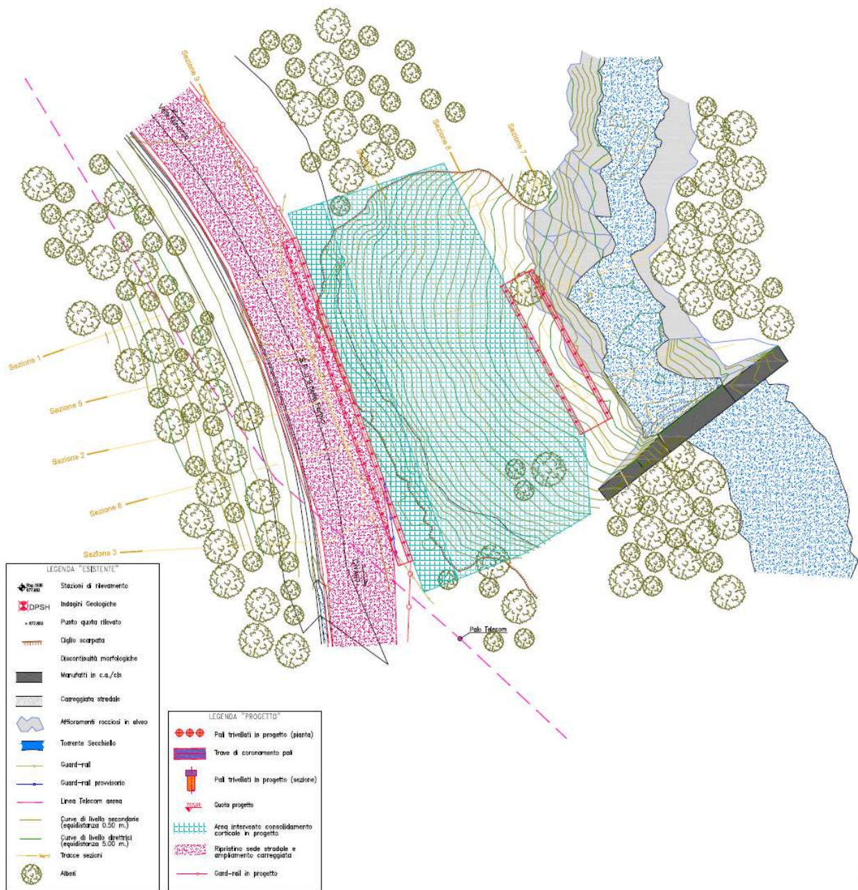
Figura 3 – Estratto della planimetria di intervento.
