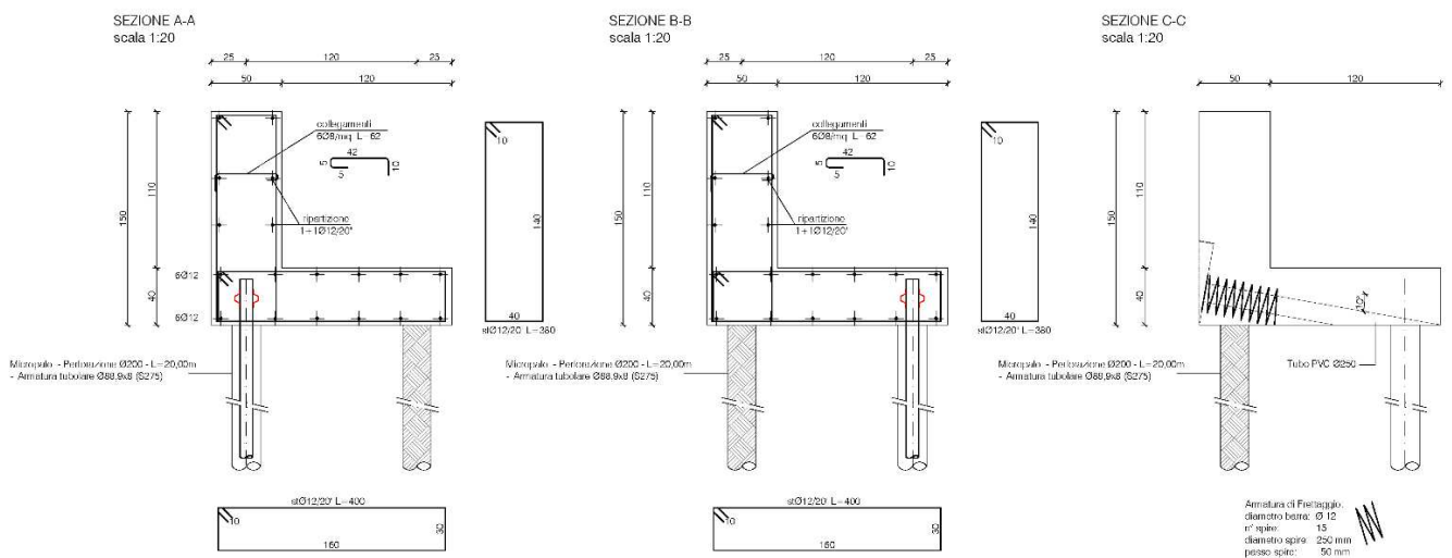
Figura 4 – Sezione tipo dei pali e della trave dell'opera di consolidamento in banchina stradale.
