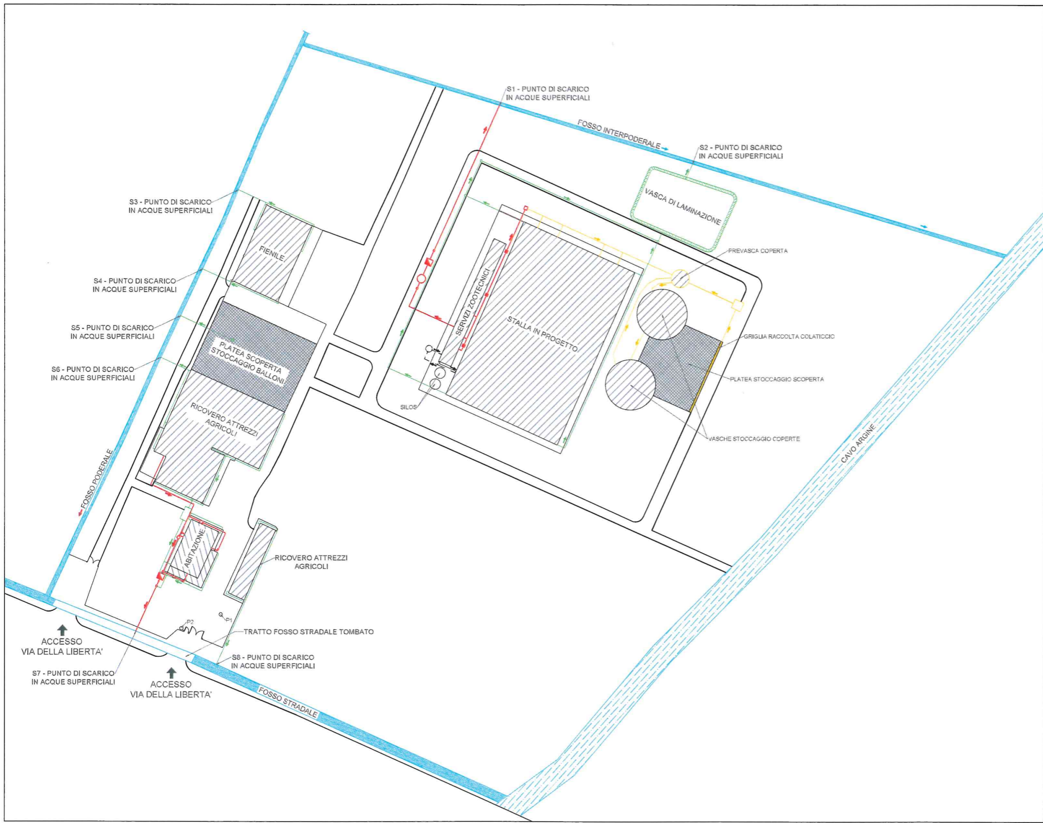
PLANIMETRIA CON INDIVIDUAZIONE PUNTI DI SCARICO IN ACQUE SUPERFICIALI - SCALA 1:1.000
