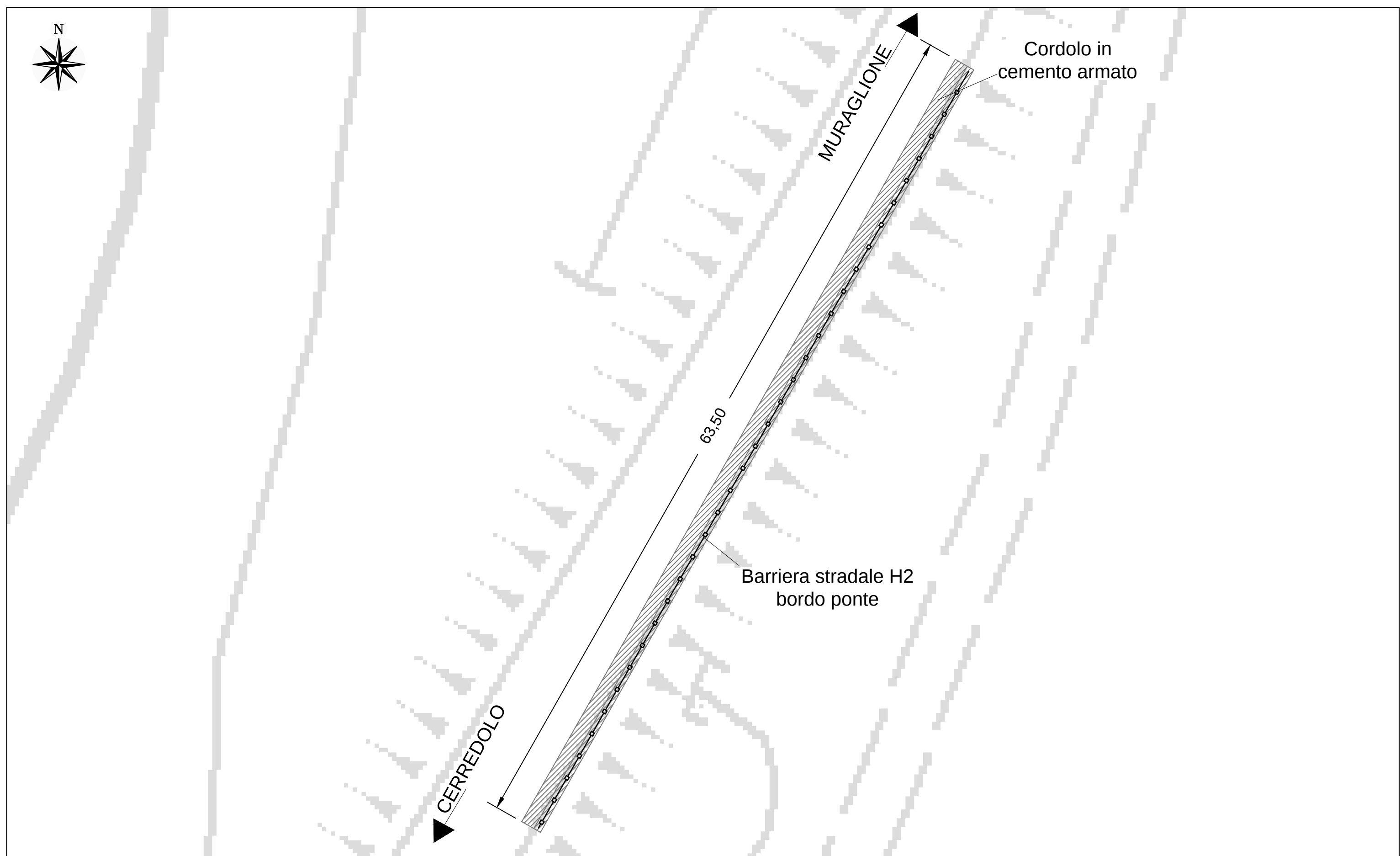
TAV.2 - INQUADRAMENTO TERRITORIALE - Lavori SP 486R km 34+050 - Scala 1:250
